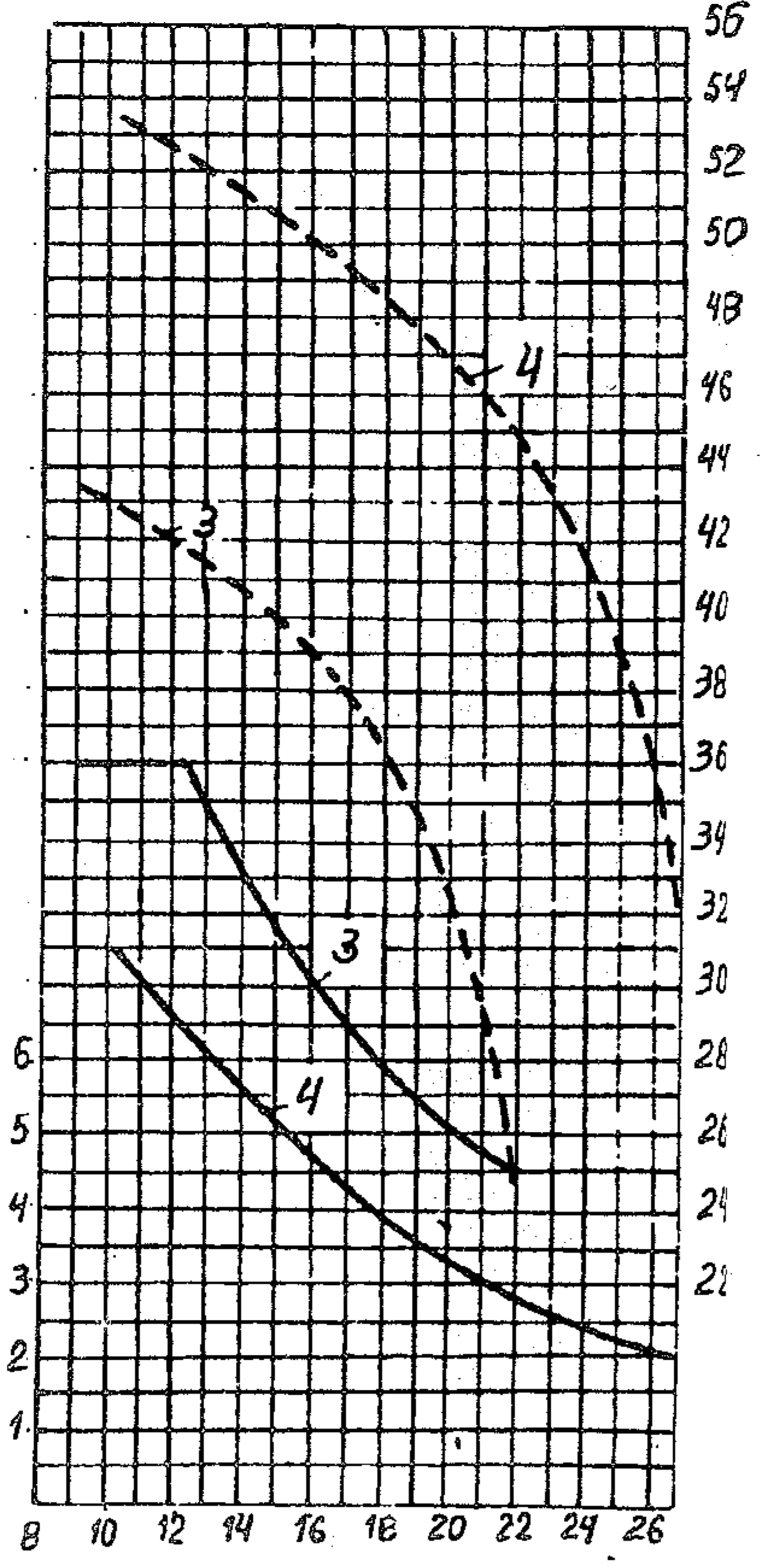
1;2;3- Tương ứng với l = 10,7; 15,8; 20,9m; L = 25m. 4- Tương ứng với l = 26m; L = 30m
