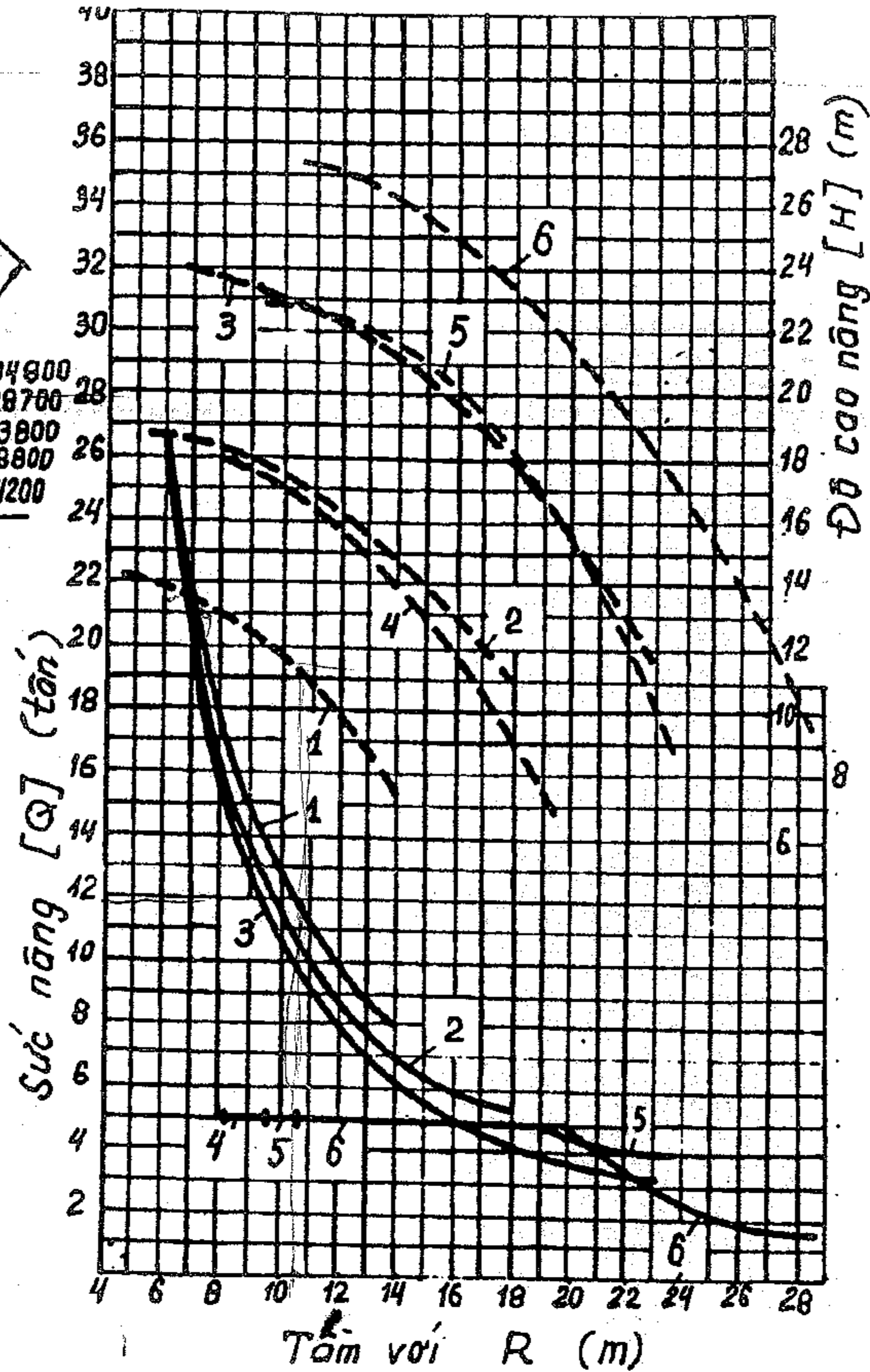
1;2;3;7;8- Móc chính, tương ứng với L = 15; 20; 25; 30 và 35m 4;5;6;9;10- Móc phụ, tương ứng với L = 15; 20; 25; 30 và 35m
