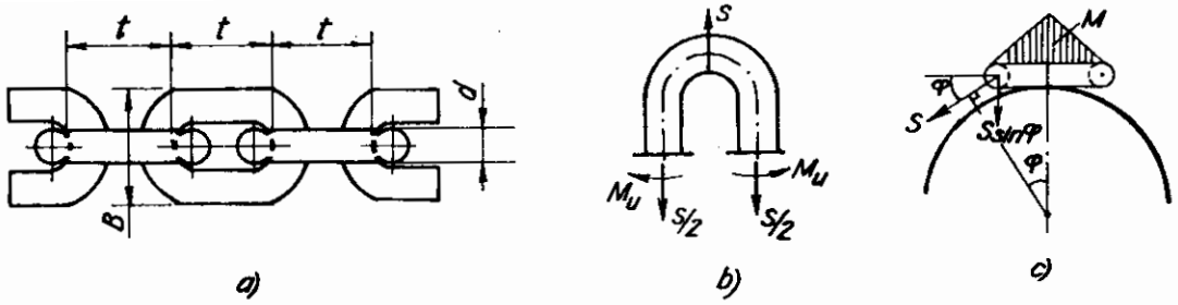
Hình 3.22: Xích hàn
