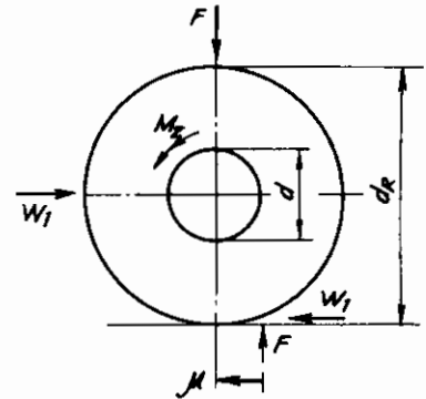
Hình 4.15: Mô hình tính lực cản ma sát.
