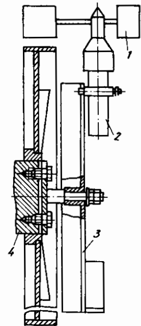
Hình 5.16: Thiết bị đo gió
