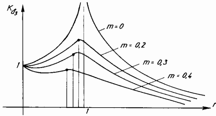
Hình 7.14: Sự phụ thuộc K_{d3} vào r .
