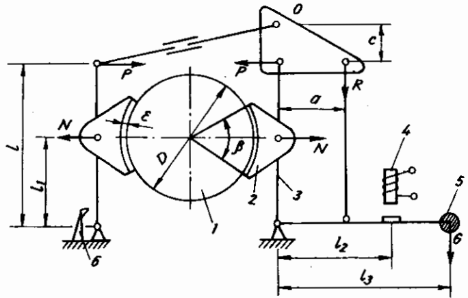
Hình 3.30: Phanh má kiểu đối trọng
