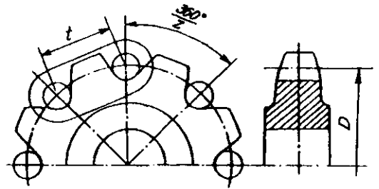
Hình 3.27: Đĩa xích dùng cho xích bản lề
