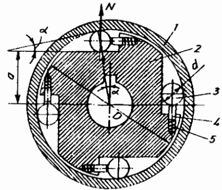
Hình 3.29: Thiết bị dùng con lăn
