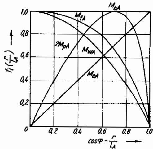
Hình 4.52: Sự phụ thuộc của các mômen vào tâm với
