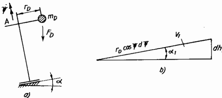
Hình 4.47: Sơ đồ tính mômen cản dốc M_\alpha
