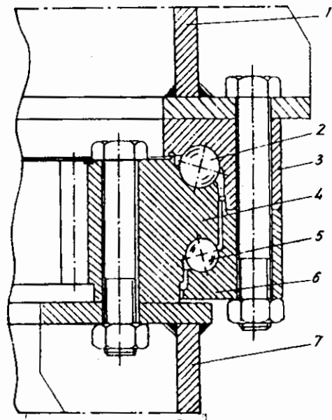
Hình 3.64: Vòng tựa quay kiểu ổ bi cầu hai dây: 1. Mặt tựa trên; 2. Dây bi đỡ; 3. Vòng đỡ; 4. Vòng cố định (có vành răng); 5. Dây bi giữ; 6. Vòng giữ; 7. Mặt tựa dưới (bệ đỡ).
