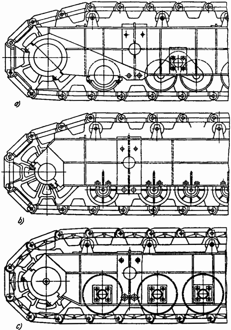
Hình 4.38: Các phương án liên kết giữa khung di chuyển và các bánh tì a) Lắp thông qua cầu cân bằng; b) Lắp trực bánh tì thông qua gối đỡ; c) Lắp trực tiếp trực bánh tì vào khung di chuyển
