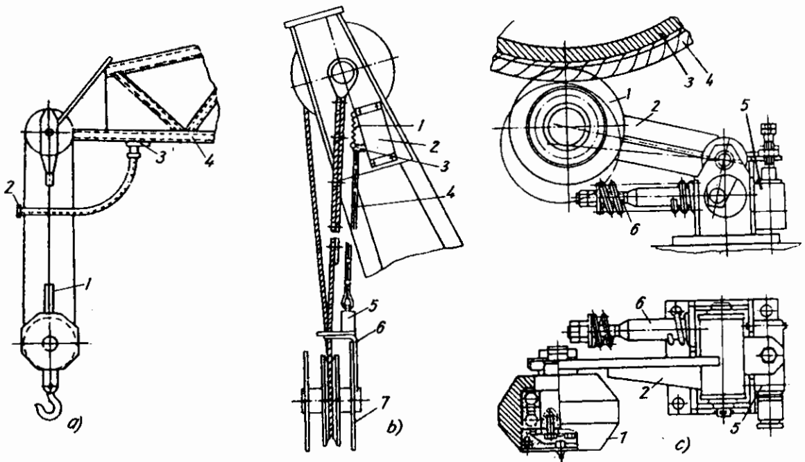
Hình 5.2: Thiết bị giới hạn chiều cao nâng a) Kiểu tay đòn; b) Kiểu cáp treo; c) Giới hạn độ sâu hạ móc treo.
