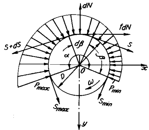
Hình 3.34: Sơ đồ lực tác dụng của đai lên bánh phanh
