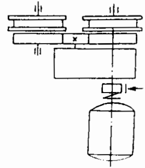
Hình 4.13: Sơ đồ cơ cấu di chuyển với hai bánh dẫn trên một cụm bánh xe
