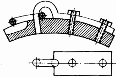
Hình 3.24: Cơ định đầu xích hàn trên tang
