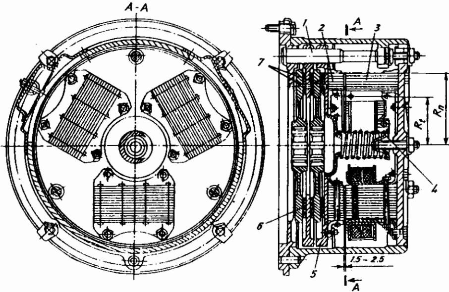
Hình 3.41: Phanh đĩa
