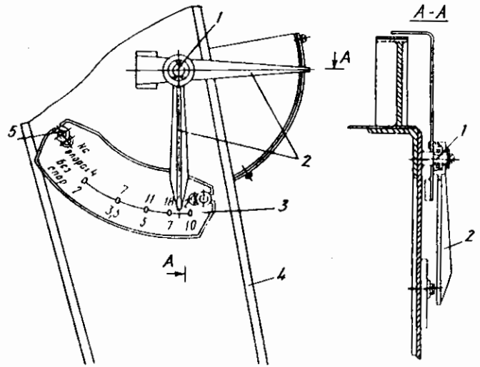
Hình 5.14: Thiết bị chỉ báo tải trọng nâng
