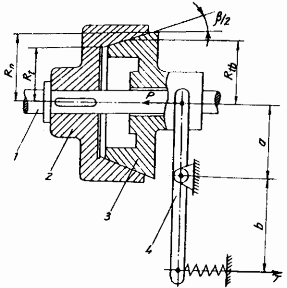
Hình 3.40: Sơ đồ tính toán phanh nón
