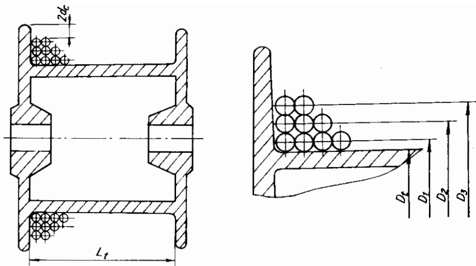
Hình 3.13: Tang nhiều lớp cáp
