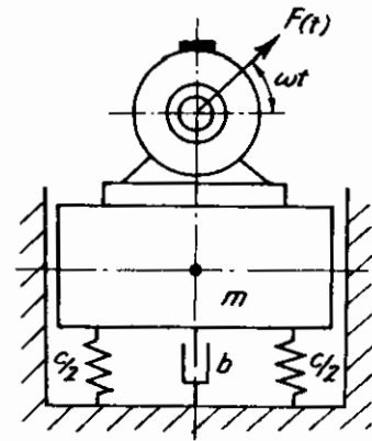
Hình 7.4: Dao động cưỡng bức một bậc tự do
