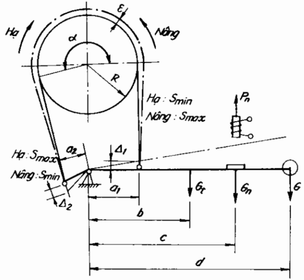
Hình 3.37: Phanh đai vi sai
