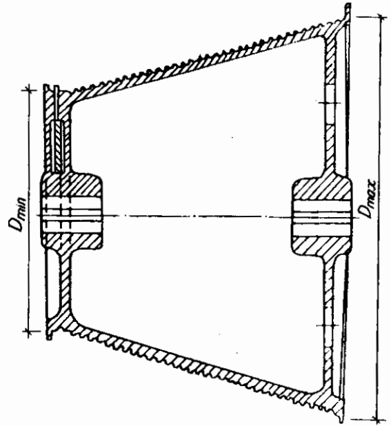
Hình 3.19: Tang côn
