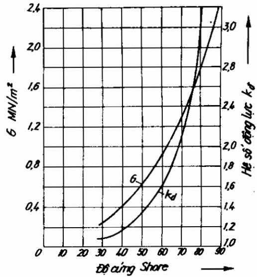
Hình 6.5: Sự phụ thuộc của môđun trượt và hệ số động lực vào độ cứng Shore
