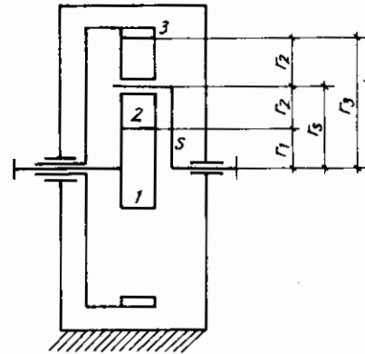
Hình 2.12: Sơ đồ nguyên lí của bộ truyền hành tinh
