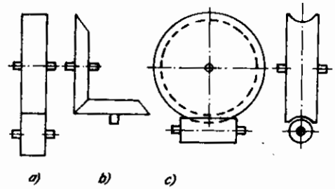
Hình 2.8: Các dạng bộ truyền ăn khớp a) Bộ truyền bánh răng trụ; b) Bộ truyền bánh răng nón; c) Bộ truyền trục vít bánh vít.
