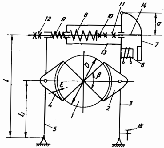
Hình 3.31: Phanh má điện từ hành trình nhỏ
