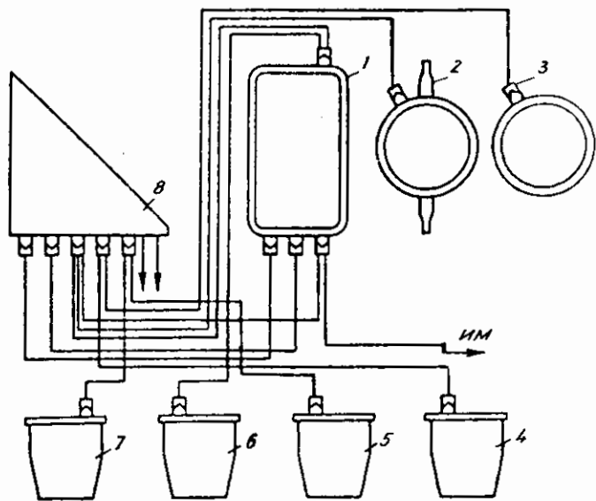
Hình 5.10: Sơ đồ nguyên lí của thiết bị giới hạn mômen tải trọng trên cần trục thủy lực với cần hộp ống lồng.
