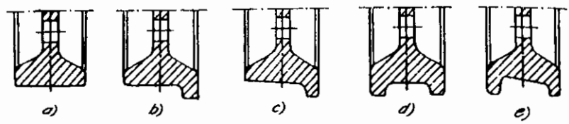
Hình 3.69: Các loại bánh xe di chuyển trên ray
