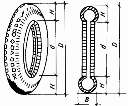
Hình 4.25: Cấu tạo và kích thước cơ bản của lốp B: Chiều rộng; D: Đường kính ngoài; d: Đường kính trong; H: Chiều cao
