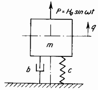
Hình 7.13: Dao động cưỡng bức có cản
