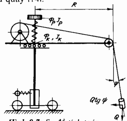
Hình 9.7: Sơ đồ tính toán động lực học cơ cấu quay
