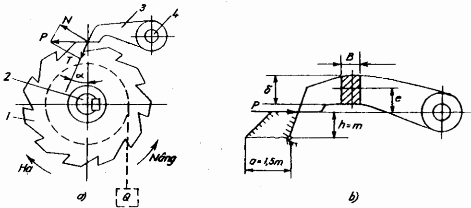
Hình 3.28: Thiết bị dừng bánh cóc
