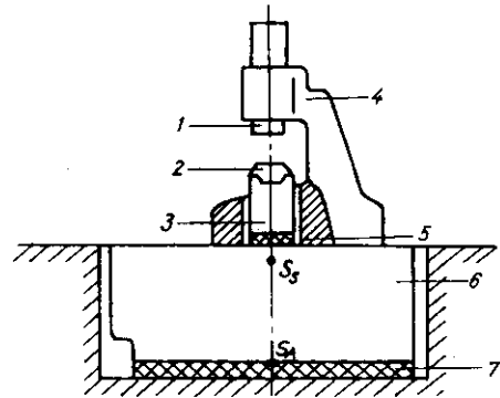
Hình 10.8: Sơ đồ lắp đặt búa máy trên móng 1. Đầu búa; 2,3. Đe và vật rèn; 4. Thân búa; 5. Đệm đàn hồi; 6. Móng khối; 7. Đệm đàn hồi; S_A, S_S - trọng tâm của diện tích đáy móng và của toàn hệ
