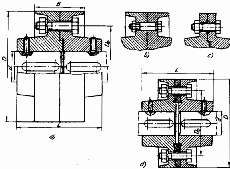
Hình 3.46: Khớp nối trực chặt kiểu đĩa
