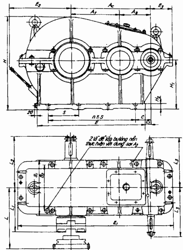
Hình 2.9: Hộp giảm tốc kiểu bánh răng trụ hai cấp
