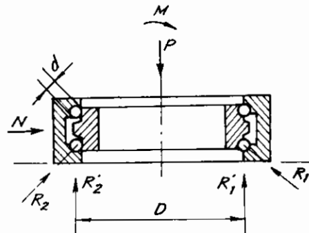
Hình 3.66: Sơ đồ tính vòng tựa quay kiểu ổ bi cầu hai dãy
