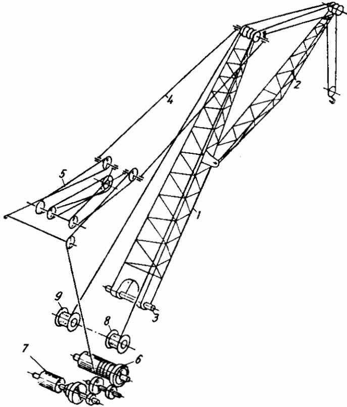
Hình 4.49: Cấu tạo chung cơ cấu nâng hạ cân
