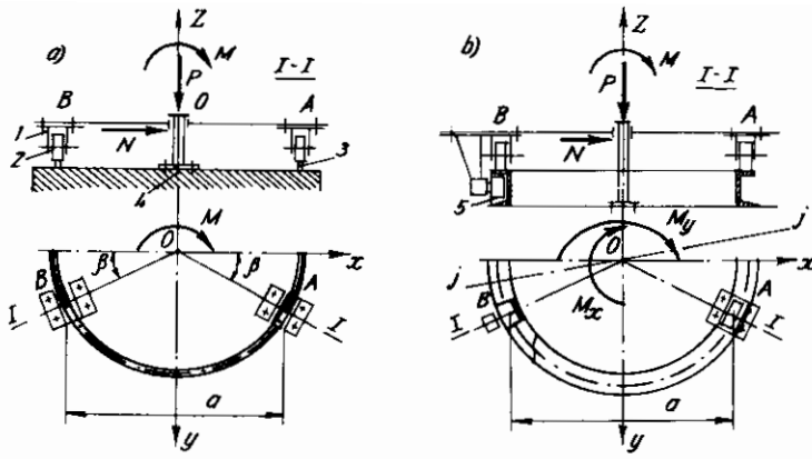
Hình 3.59: Vòng tựa quay kiểu bánh tựa
