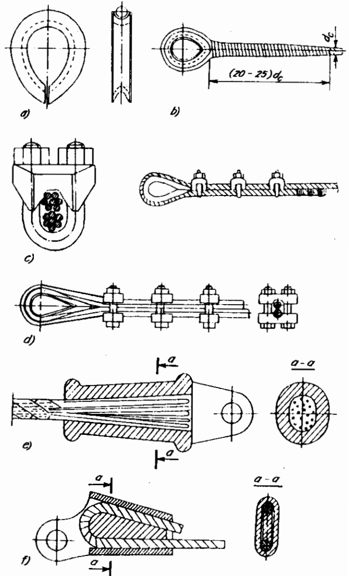
Hình 3.4: Các phương pháp cố định đầu cáp với trục
