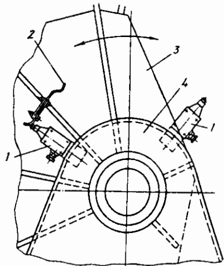
Hình 5.5: Thiết bị giới hạn góc nghiêng cần
