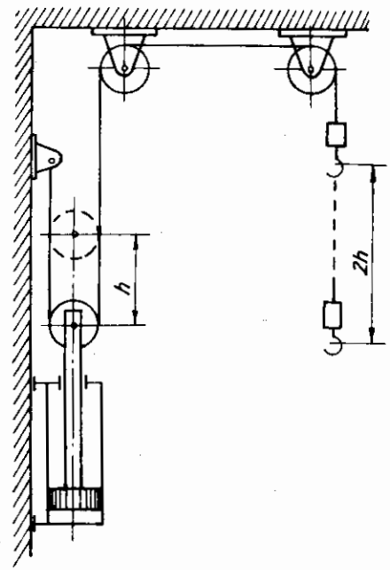
Hình 3.9: Palăng vận tốc
