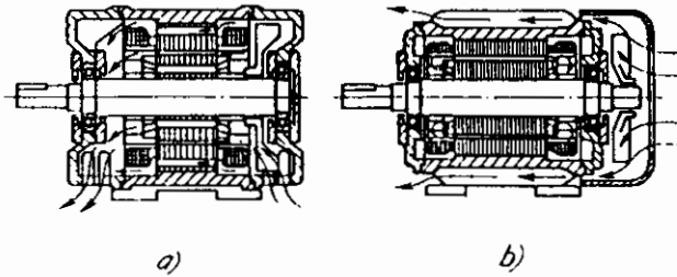
Hình 2.3: Động cơ tự làm mát
