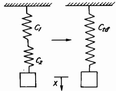
Hình 6.4: Hệ hai lò xo mắc nối tiếp
