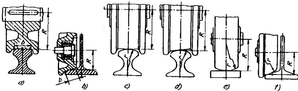
Hình 3.73: Các phương án phối hợp hình dạng bánh xe và ray
