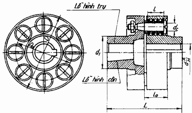
Hình 3.50: Khớp nối đàn hồi có ống lót cao su
