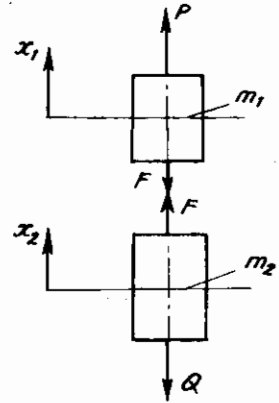
Hình 9.4: Mô hình tính toán cơ cấu nâng 2 bậc tự do
