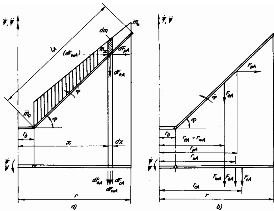
Hình 4.44: Lực tác dụng lên cần khi quay quanh trục đứng a) Các lực phân tử; b) Lực và bán kính quy đổi
