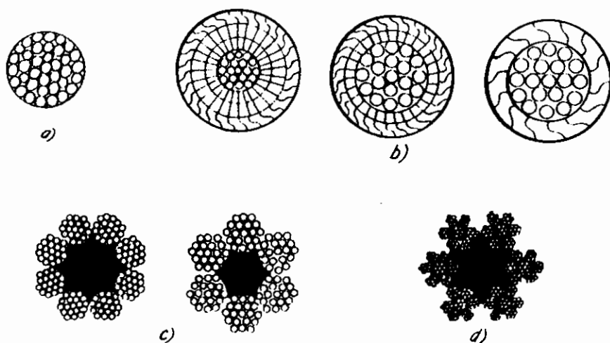
Hình 3.1: Các loại cáp thép theo số lớp bện
