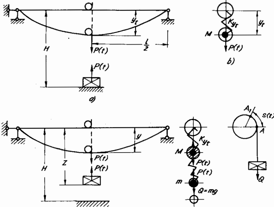
Hình 9.5: Quá trình động lực học khi nâng vật nằm trên nền cứng.
