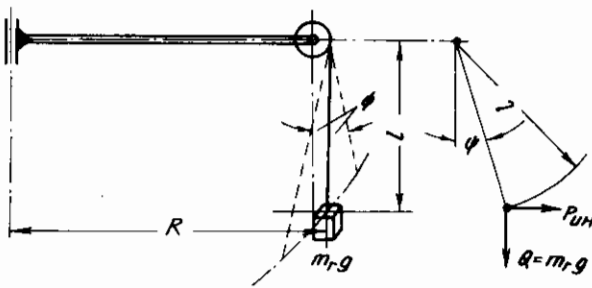
Hình 9.6: Sơ đồ tính toán góc nghiêng \psi của tải trọng khi quay
