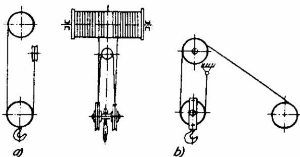
Hình 4.2: Sơ đồ mắc cáp cơ cấu nâng a) Vật nặng treo trực tiếp dưới tang; b) Vật nặng treo thông qua puli đối hướng cáp.
