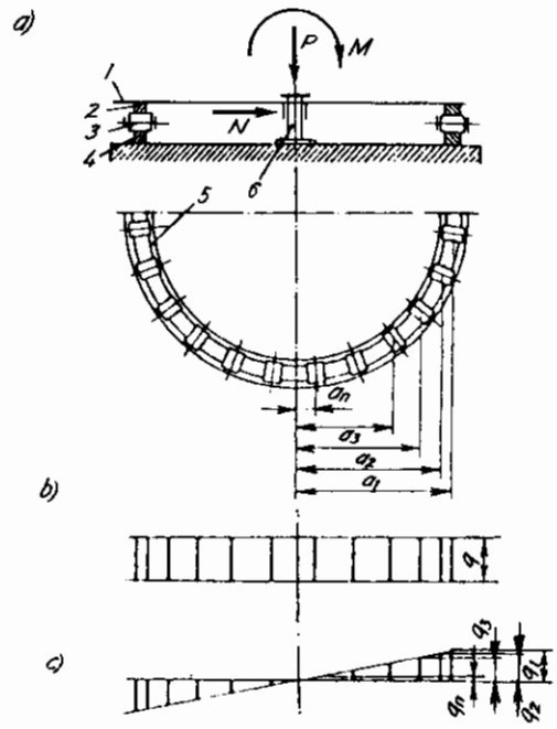
Hình 3.63: Sơ đồ tính vòng tựa quay kiểu con lăn
