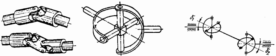
Hình 3.49: Khớp cacđăng
