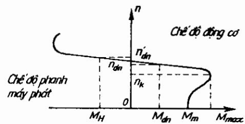
Hình 2.4: Đặc tính cơ của động cơ lồng sóc
