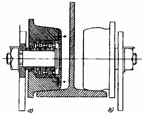
Hình 3.71: Bánh xe của xe con chạy trên ray treo
