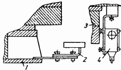
Hình 5.4: Thiết bị giới hạn góc quay
