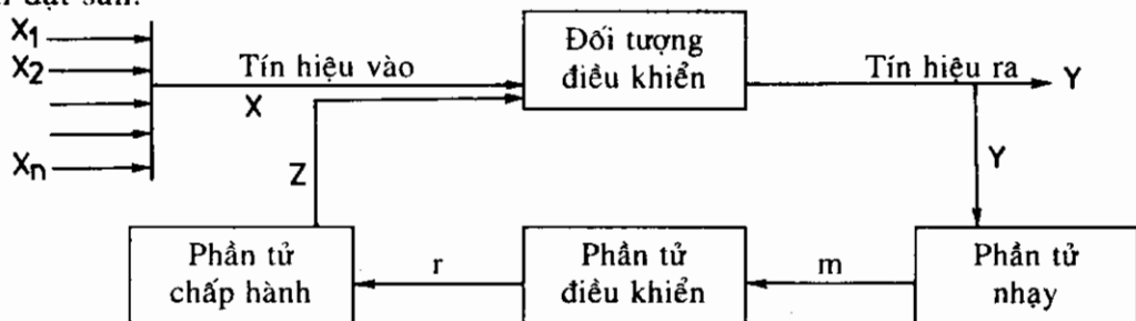
Hình 5.23: Sơ đồ nguyên lí hệ thống điều khiển tự động mạch kín
