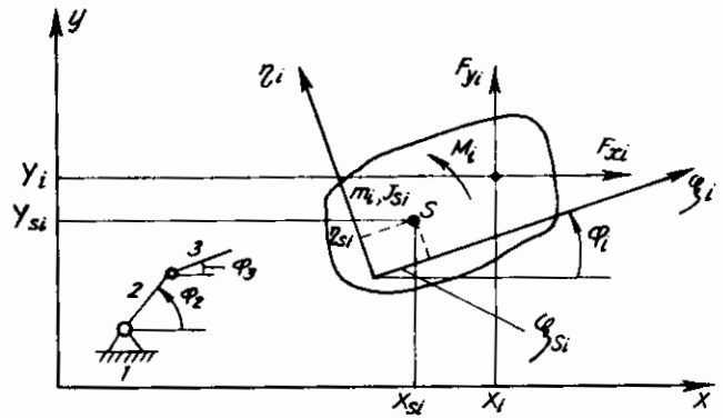
Hình 8.1: Khâu có chuyển động phẳng
