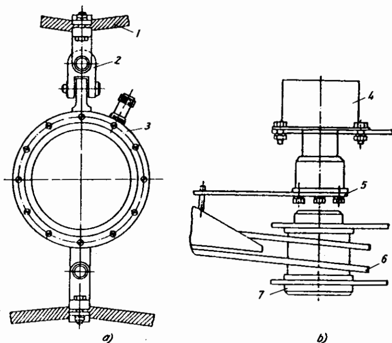
Hình 5.9: Thiết bị giới hạn mômen tải trọng a) Bộ cảm biến lực; b) Bộ cảm biến góc nghiêng cân.
