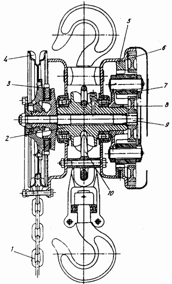
Hình 2.16: Pa lăng xích với truyền động bánh răng hành tinh
