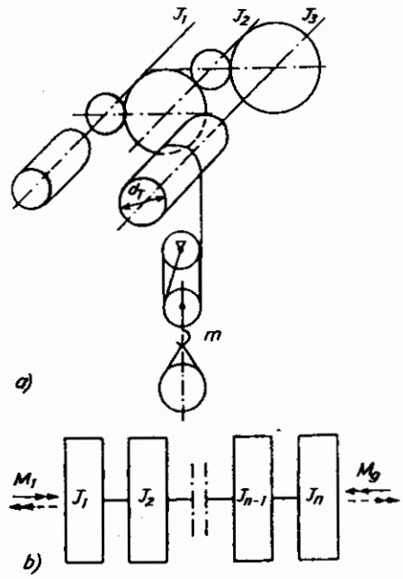
Hình 4.7: Sơ đồ cơ cấu nâng a) Các khối lượng phân bố trên các trục; b) Quy dẫn các khối lượng về trục động cơ.
