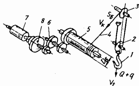
Hình 4.1: Sơ đồ cấu tạo chung của cơ cấu nâng với tời cáp 1. Móc treo; 2. Puli di động; 3. Puli cố định; 4. Cáp; 5. Tang; 6. Bộ truyền bánh răng (hộp giảm tốc); 7. Động cơ điện; 8. Phan.
