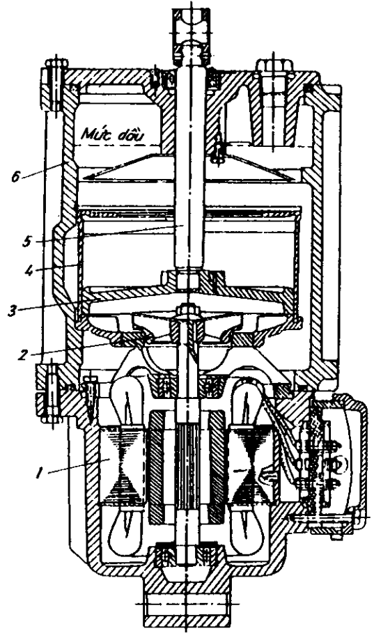
Hình 3.33: Con đẩy điện - thủy lực
