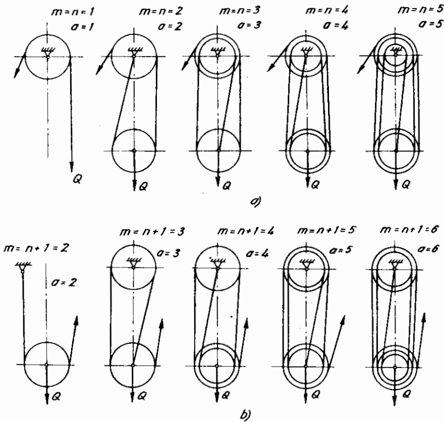
Hình 3.7: Palăng đơn
