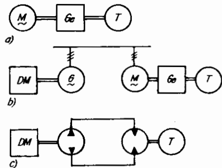
Hình 2.1: Sơ đồ hệ truyền động
