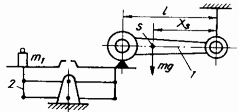
Hình 6.1: Xác định tọa độ trọng tâm bằng phương pháp tính
