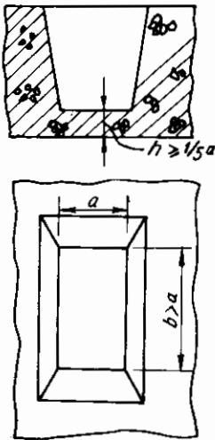
Hình 10.12: Kích thước chiều dày đáy ở trống
