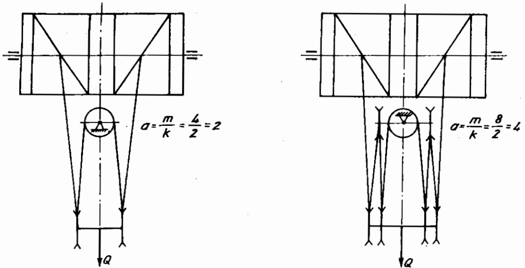
Hình 3.8: Palăng kép
