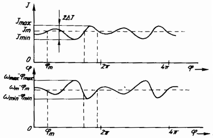
Hình 8.3: Các giai đoạn chuyển động của máy.
