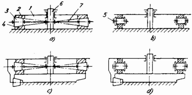
Hình 3.62: Vòng tựa quay kiểu con lăn
