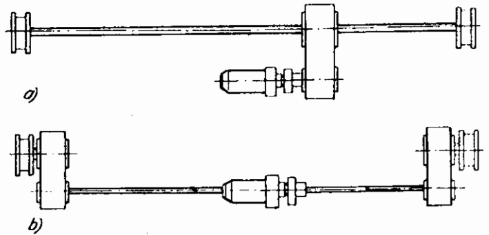
Hình 4.10: Các sơ đồ cơ cấu di chuyển dẫn động chung a) Trục truyền quay nhanh, b) Trục truyền quay chậm.
