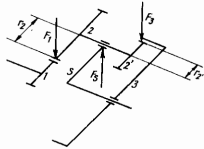
Hình 2.13: Lực trên bộ truyền hành tinh.
