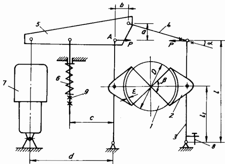
Hình 3.32: Phanh má điện - thủy lực
