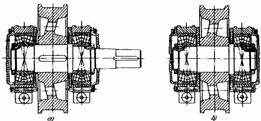
Hình 3.68: Cụm bánh xe chủ động và bị động
