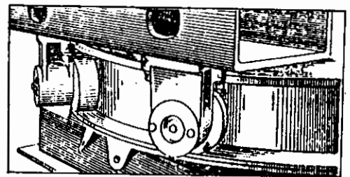
Hình 3.60: Lắp đặt các con lăn tì chống lật chịu phản lực thẳng đứng
